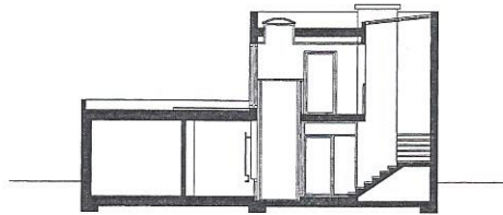
COUPE A-A'
